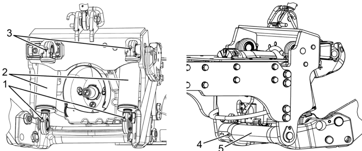
Рисунок 5.4.22 – Смазка шарниров гидроцилиндров и оси качания рамки нижних тяг ПНУ
