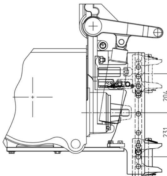
Рисунок 4.4.1 – Схема вариантов установки вилки не вращающейся
