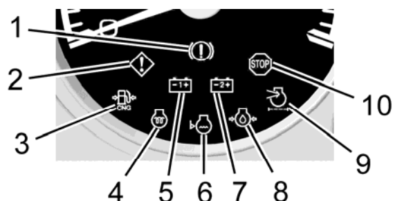
Рисунок 2.5.2 – Расположение сигнализаторов встроенных в указатель частоты оборотов коленчатого вала двигателя
