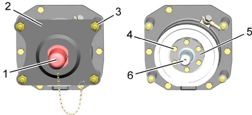
1 – колпак; 2 – плита; 3 – гайка; 4 – болт; 5 – пластина; 6 – хвостовик.
