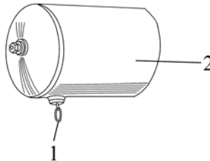
Рисунок 5.4.5 – Удаление конденсата из баллона пневмосистемы
