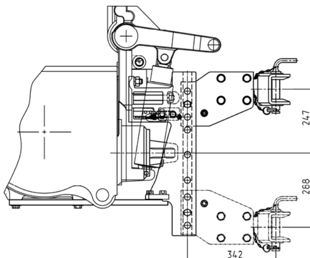
Рисунок 4.4.2 – Схема вариантов установки вилки вращающейся длиной
