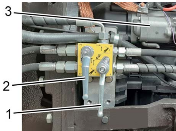
1, 2 – рукоятки крана управления ПНУ; 3 – стартер.
