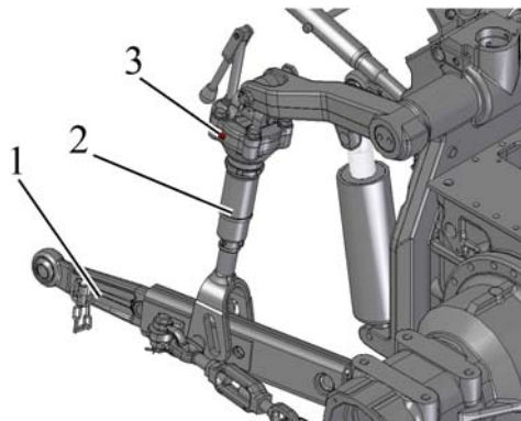
1 – нижняя тяга ЗНУ; 2 – шестеренчатый раскос; 3 – маслѐнка.
