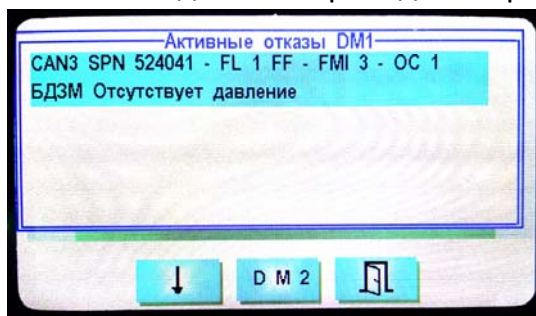
Рисунок 6.17.1 – Пример отображения ошибки на дисплее
