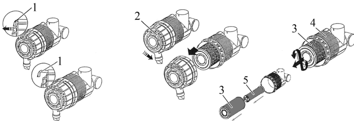
Рисунок 5.4.31 – Обслуживание воздухоочистителя двигателя
