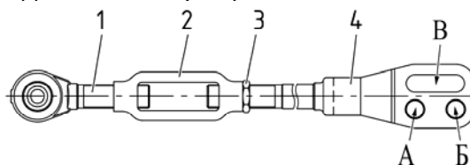
1 – винт с шарниром; 2 – стяжка; 3 – контргайка; 4 – вилка.
