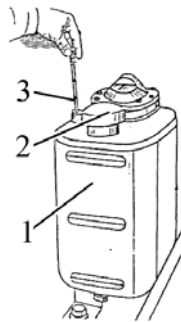
Рисунок 5.4.3 – Проверка уровня масла в баке ГОРУ
