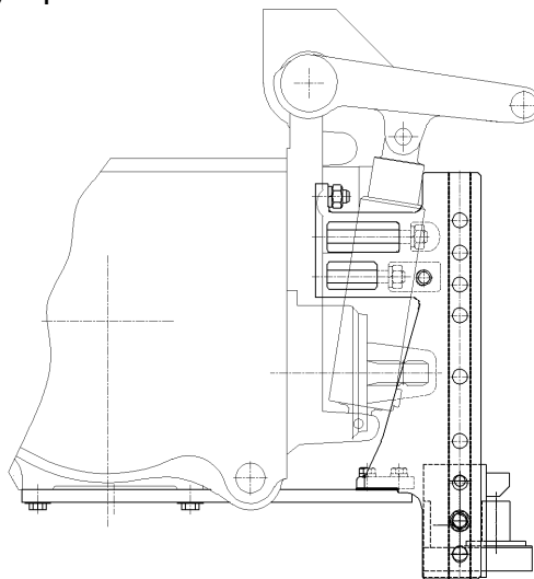
Рисунок 4.4.8 – Схема установки элемента типа «питон» по ISO 6489-4 (рекомендуемое положение)
