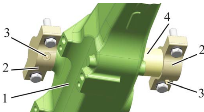
Рисунок 5.4.20 – Смазка подшипников бугелей (вид снизу ПВМ)
