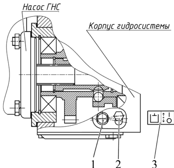
Рисунок 2.15.1 – Управление насосом ГНС
