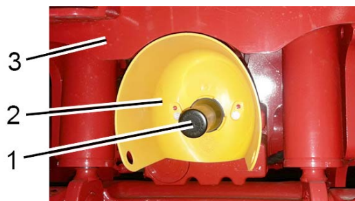
1 – колпак; 2 – защитный кожух; 3 – переднее навесное устройство.
