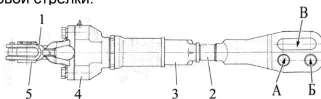
1 – рукоятка; 2 – вилка; 3 – труба; 4 – корпус; 5 – серьга.
