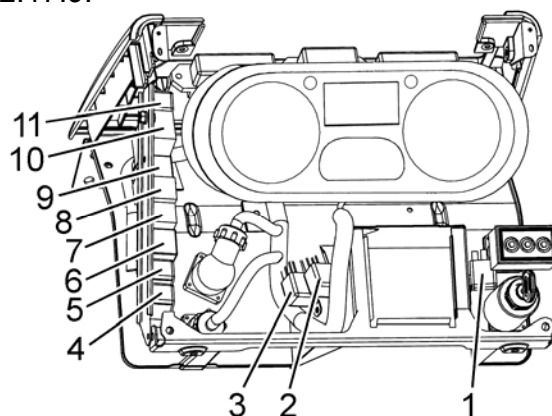
Рисунок 2.17.8 – Размещение электромагнитных реле в щитке приборов
