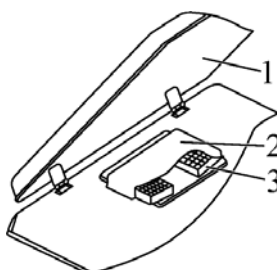
1 – крыша кабины; 2 – крышка фильтра; 3 – фильтрующий элемент.
