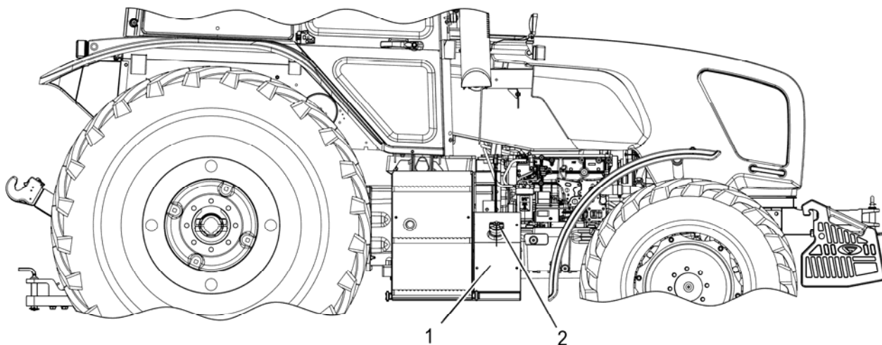
Рисунок 2.21.1 – Установка бака для жидкости системы SCR
