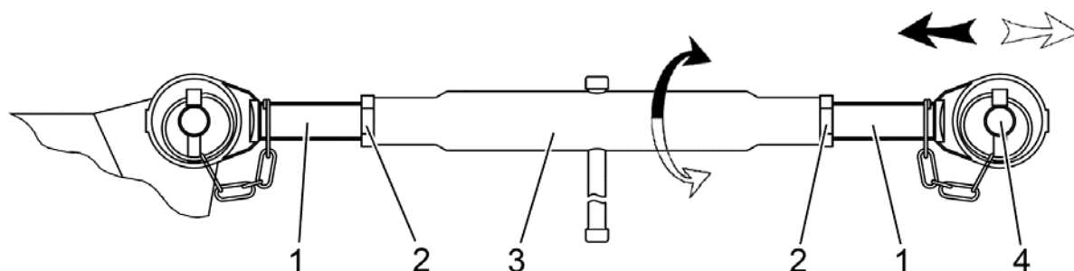
1 – винт с шарниром; 2 – контргайка; 3 – труба; 4 – палец.
