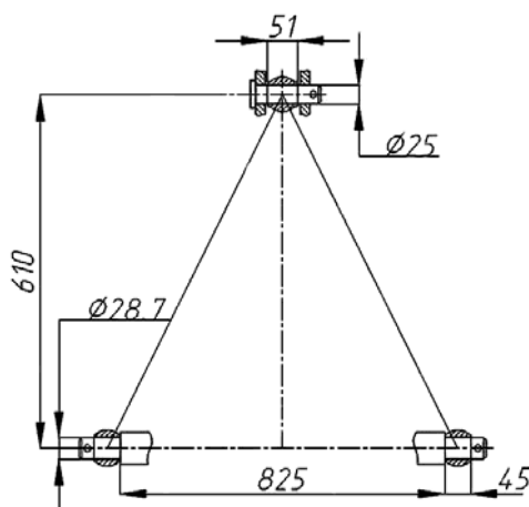
Рисунок 4.3.13 – Схема переднего навесного устройства
