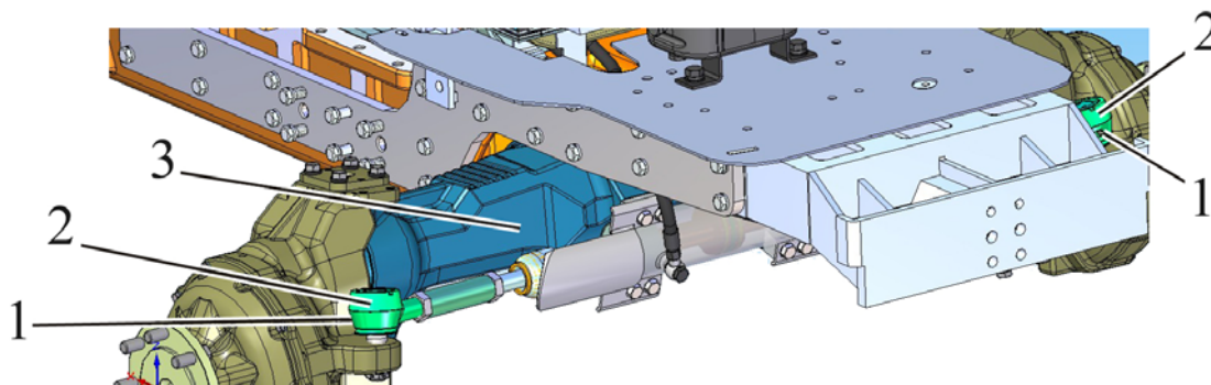
1 – масленка; 2 – шарнир рулевой тяги; 3 – ПВМ
