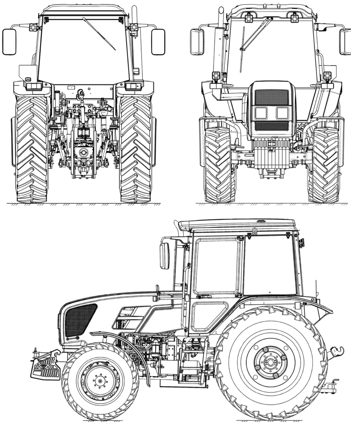
Рисунок 1.1.1 – Трактор «БЕЛАРУС-952.7» в базовой комплектации
