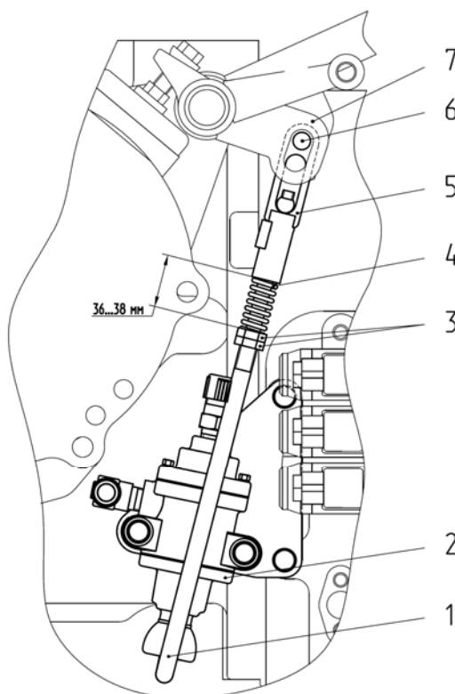
Рисунок 5.4.25 – Регулировка привода тормозного крана пневмосистемы
