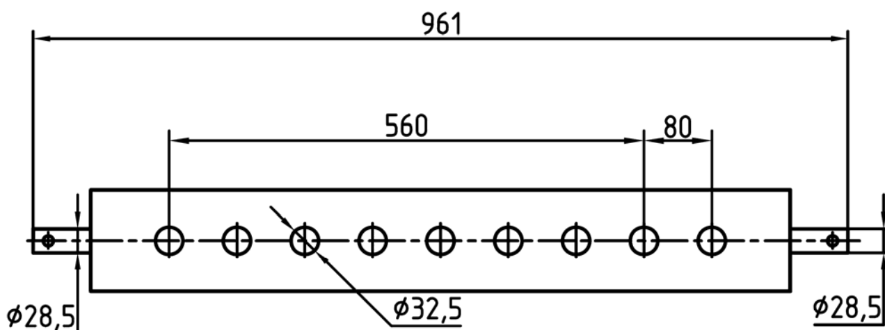
Рисунок 4.4.12 – Схема установки поперечины
