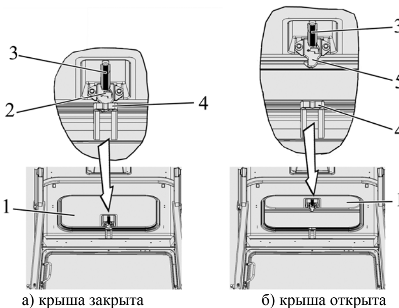
Рисунок 2.18.4 – Открытие крыши кабины
