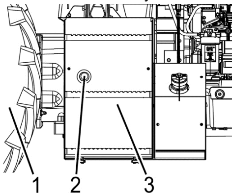
Рисунок 2.2.3 – Установка ручного выключателя АКБ
