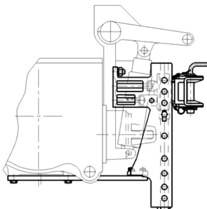
Рисунок 4.4.5 – Схема установки вилки вращающейся неавтоматической короткой (рекомендуемое положение) по ГОСТ 32774 и ISO 6489-2
