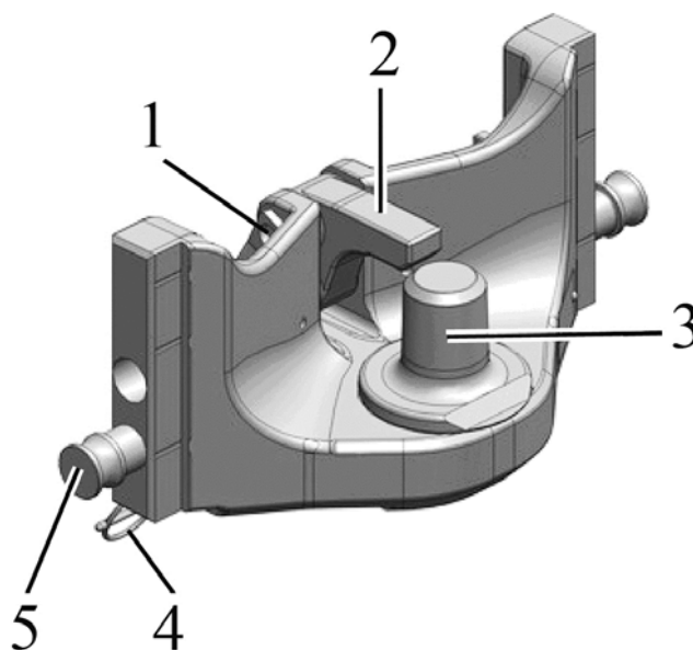
Рисунок 4.4.9 – Элемент ТСУ типа «питон» по ISO 6489-4
