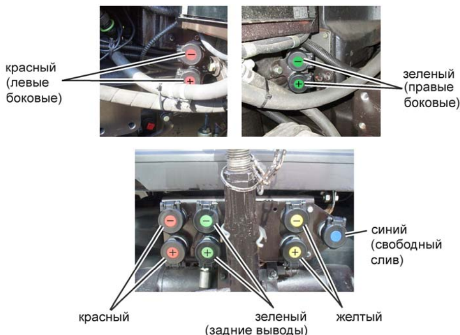
Рисунок 2.16.3 – Расположение и подключение выводов распределителя к внешним потребителям
