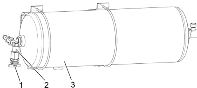
1 – гайка-барашек; 2 – клапан контрольного вывода; 3 – баллон пневмосистемы.
