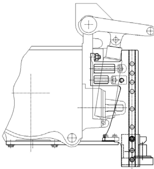
Рисунок 4.4.10 – Схема установки элемента типа «питон» нестандартный (рекомендуемое положение)
