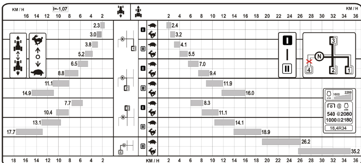
Рисунок 2.11.2 – Диаграмма скоростей трактора «БЕЛАРУС-952.7»
