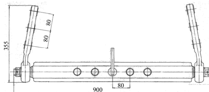
Рисунок 4.4.13 – Схема установки двойной поперечины
