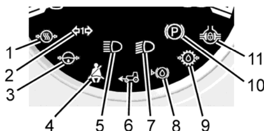
Рисунок 2.5.3 – Расположение сигнализаторов встроенных в указатель скорости
