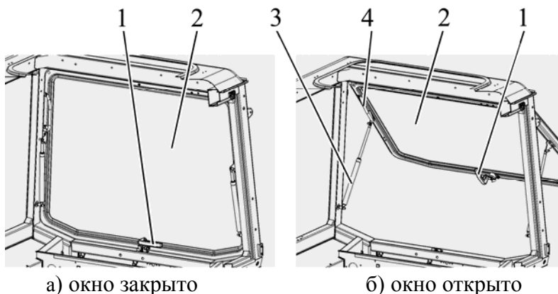
Рисунок 2.18.3 – Открытие заднего окна
