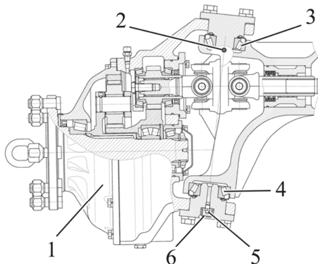
Рисунок 5.4.19 – Смазка подшипников осей шкворней ПВМ
