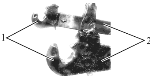
1 – захват; 2 – тяга.
