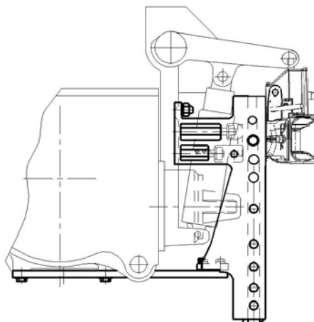
Рисунок 4.4.6 – Схема установки вилки вращающейся автоматической по ISO 6489-2 (рекомендуемое положение)
