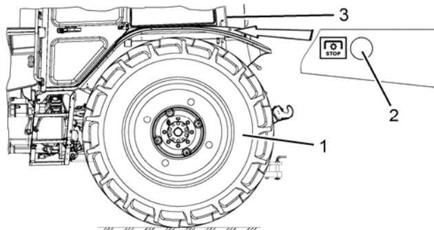
1 – заднее колесо; 2 – кнопка выключения привода ЗВОМ; 3 – заднее стекло кабины.
