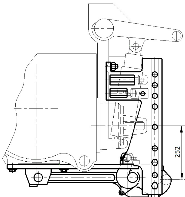
Рисунок 4.4.3 – Смонтированный тяговый крюк
