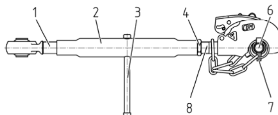
б) верхняя тяга с захватом
