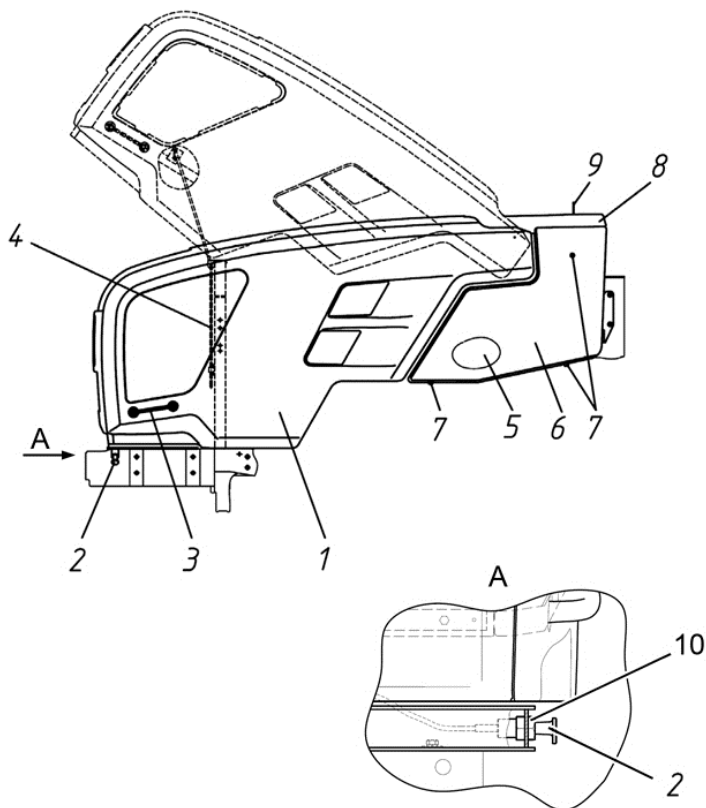
Механизм открытия капота и его фиксации в открытом положении
