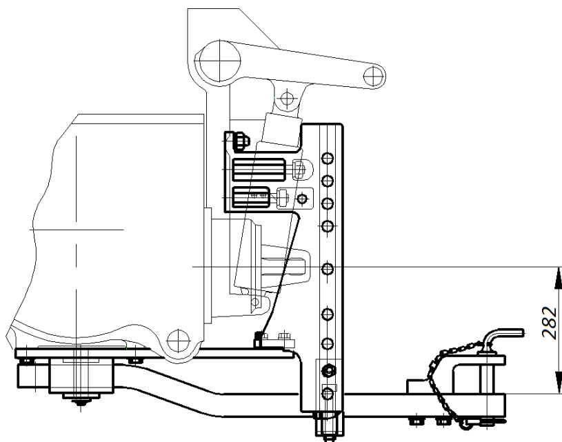
Рисунок 4.4.11 – Тяговый брус
