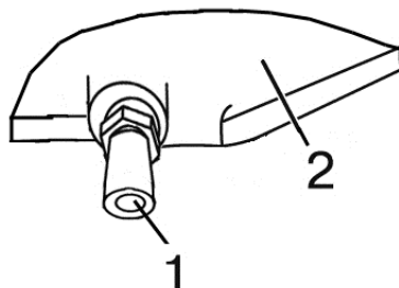
1 – штуцер; 2 – топливный бак.
