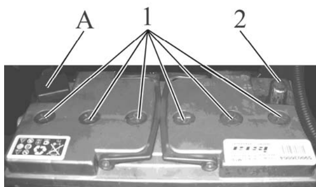
Рисунок 7.3.2 – Обслуживание аккумуляторных батарей
