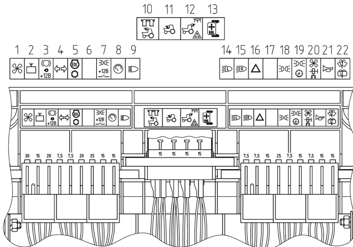
Рисунок 2.17.2 – Размещение предохранителей в щитке приборов
