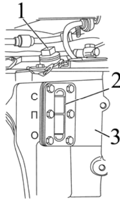
Рисунок 5.4.2 – Проверка уровня масла в баке ГНС
