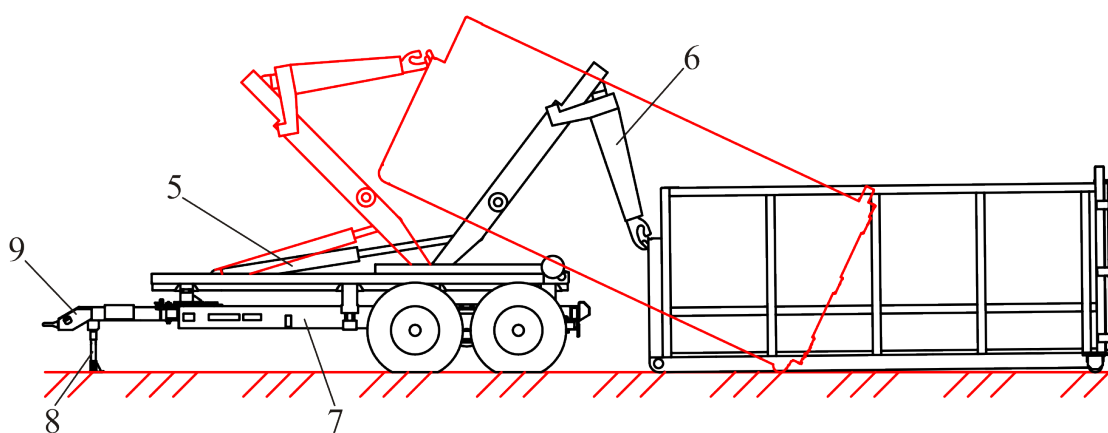
б) Вид полуприцепа при разгрузке мультитрифтовым способом
