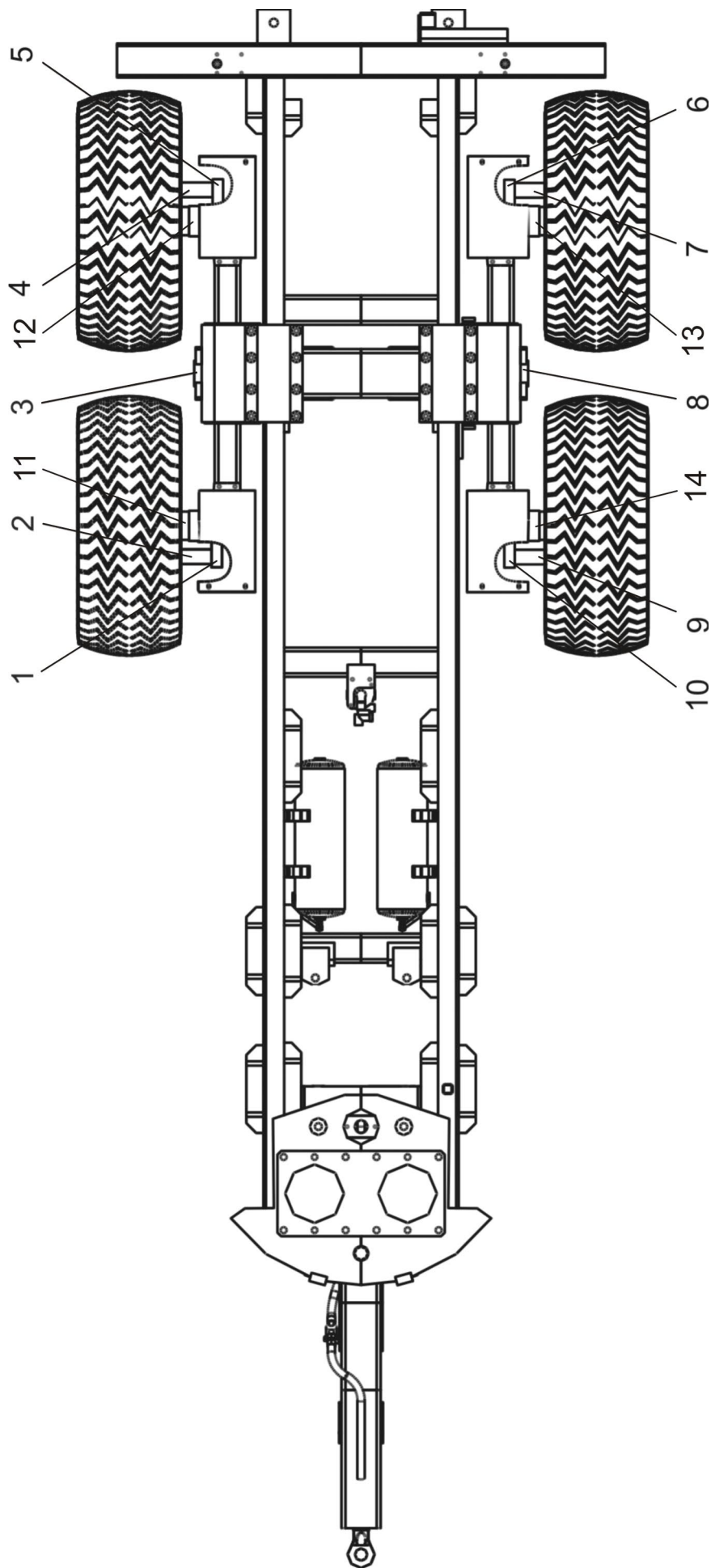
1, 5, 6, 10 – тормозные рычаги; 2, 4, 7, 9 – валы разжимных кулаков; 3, 8 – оси балансиров; 11, 12, 13, 14 – подшинниковые узлы колес
