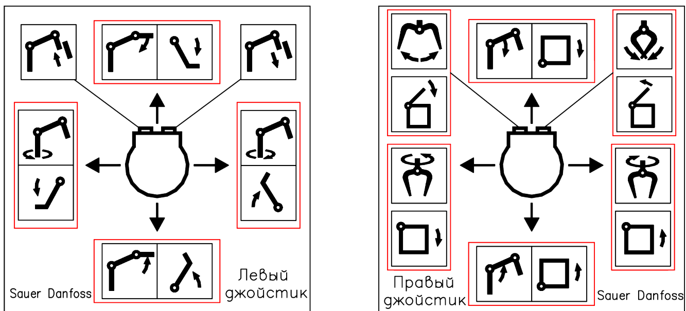
Рисунок 17 – Схема управления гидроманипулятором, аутригерами и бункером
