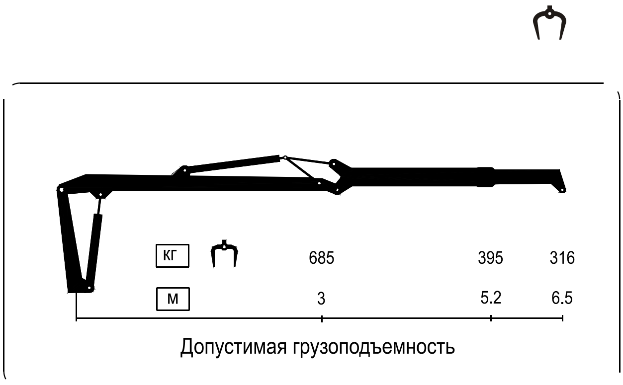
Рисунок 19 – Табличка грузоподъемности гидроманипулятора ГМ-42Т-01
