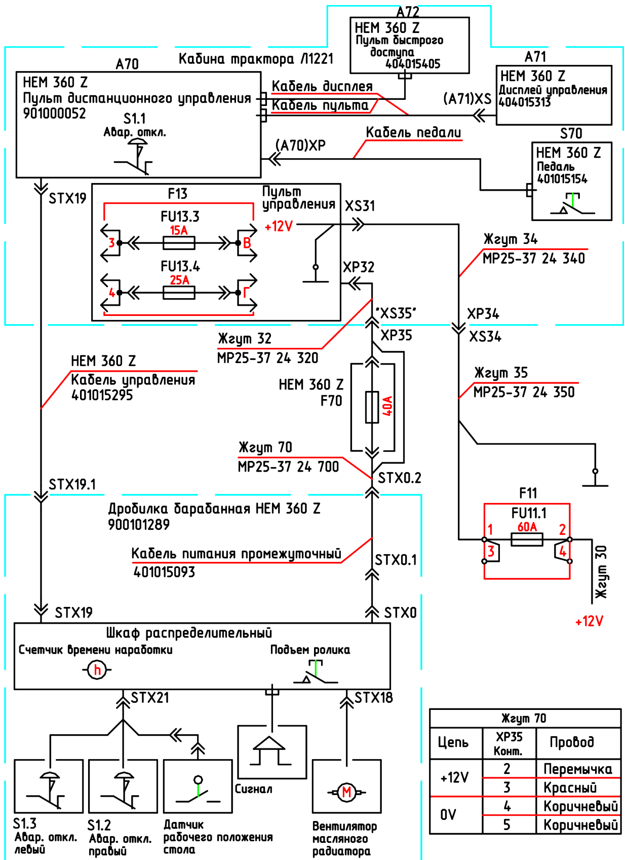
Рисунок 13 – Схема электрическая соединений электрооборудования рубильного агрегата
